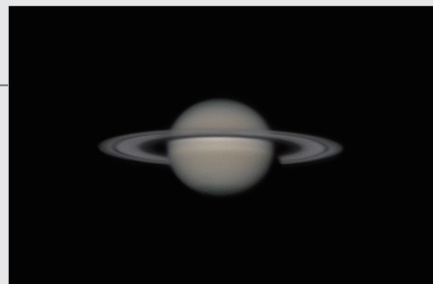
「土星」(2026 年 8 月 13 日撮影) 撮影者: 渡辺文健
